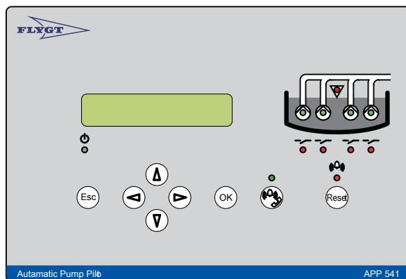
Светодиодные индикаторы на панели оператора
